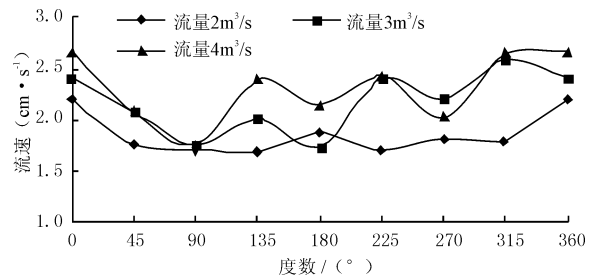
图9 曲线二型中心出水环堰不同流量下溢流堰的行近流速分布图
