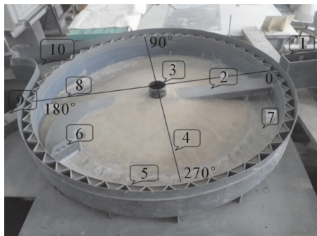
1 - 进水渠; 2 - 进水廊道; 3 - 中心出水环; 4 - 倒锥底坡; 5 - 迷宫型溢流堰; 6 - 环流闸; 7 - 冲沙槽; 8 - 冲沙廊道; 9 - 冲沙闸; 10 - 出水渠
