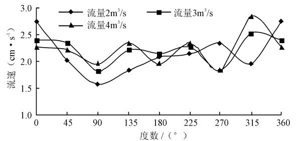
图8 曲线一型中心出水环堰不同流量下溢流堰的行近流速分布图
