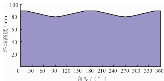
图 2 曲线型中心出水环堰展开图
