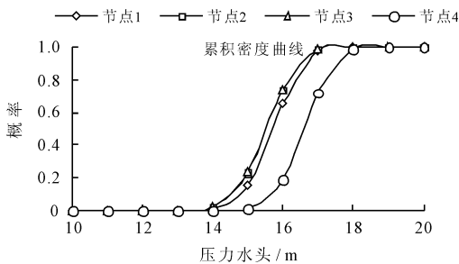
图 4 节点测压管水头的累积密度函数曲线图
