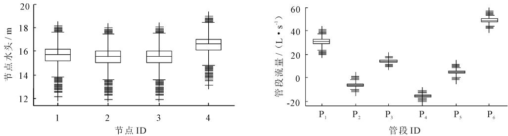
图 3 管网测压管水头和管段流量的箱型图
