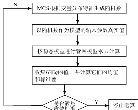
图1 算法流程图
