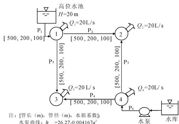
图2 管网拓扑图
