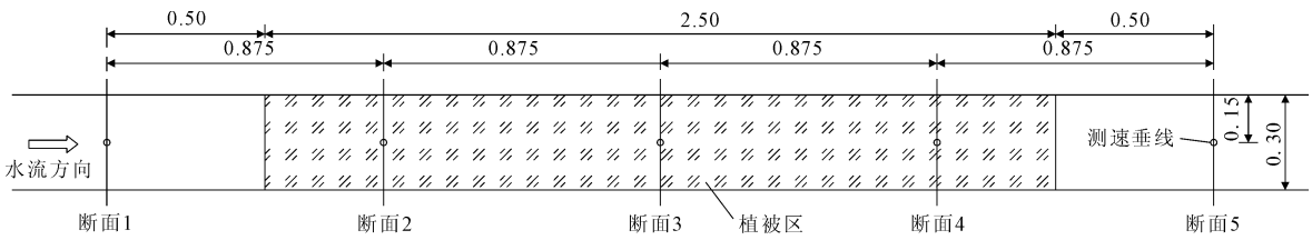
图 1 测点平面布置图(单位:m)
